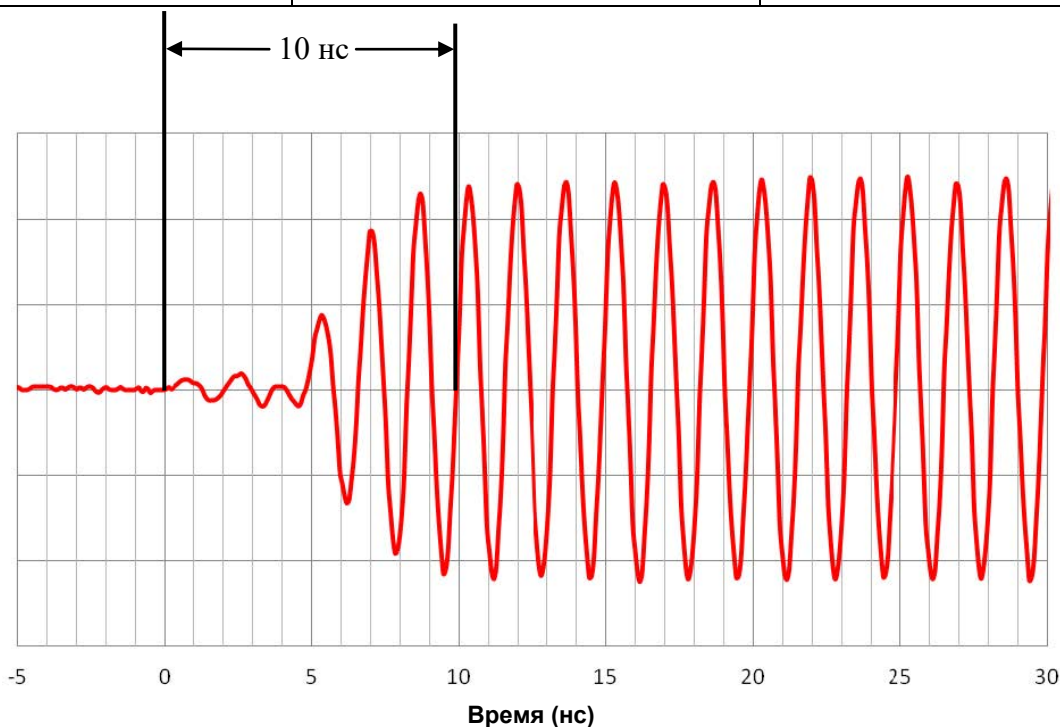
Рисунок 20: Время нарастания внешней импульсной модуляции (секунды)
