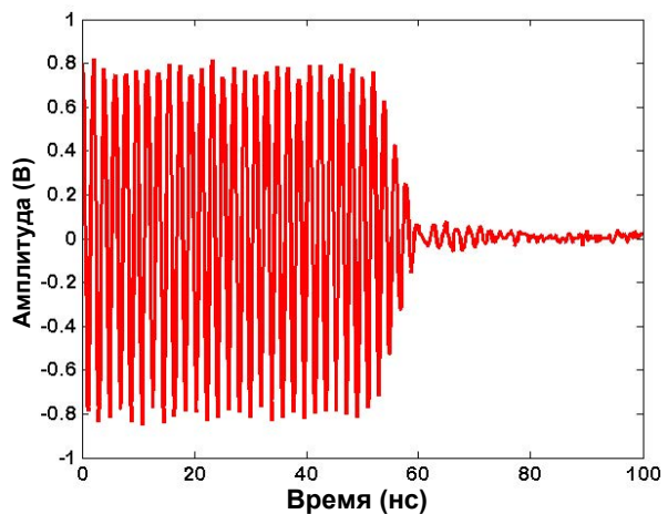
Рисунок 19б: Время нарастания импульсной модуляции, f_c = 530 МГц
