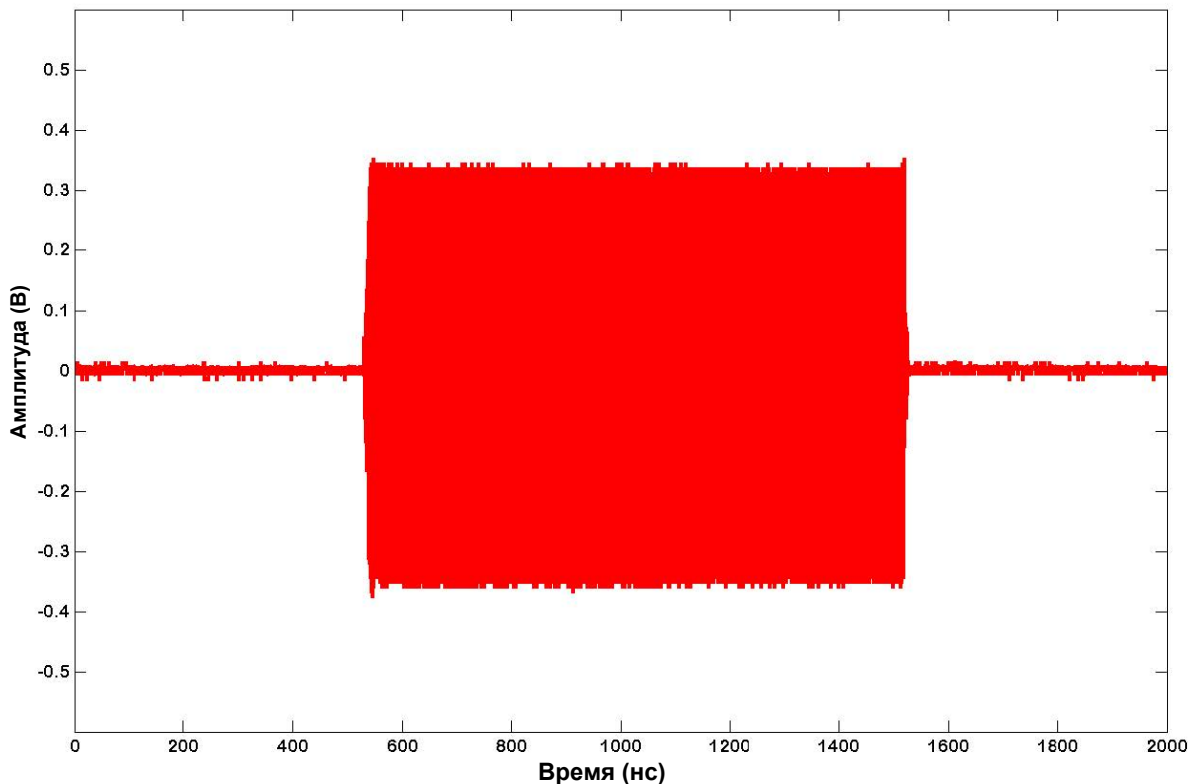
Рисунок 17: Частота внутренней импульсной модуляции f_c = 500 МГц, Импульс 2 нс 2
